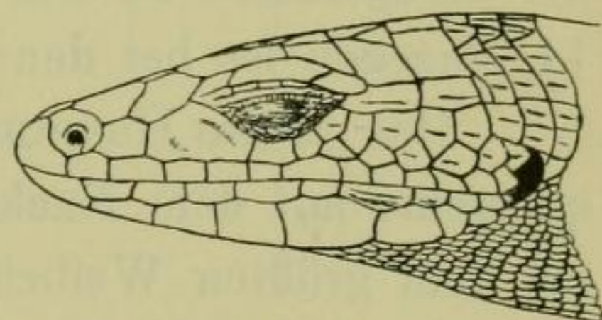
Fig. 1. Zonurus pustulatus .
