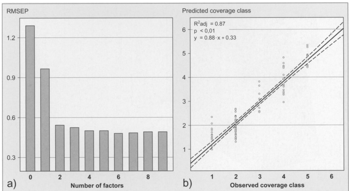
Fig. 2: a) Root-mean-square-error of prediction (RMSEP) in relation to the number of latent factors (RMSEP Min for n = 6 ); b) Woody coverage predicted by PLSR ( n = 6 ) in relation to woody coverage observed in the field a) Mittlerer quadratischer Vorhersagefehler in Abhängigkeit von der Anzahl latenter Faktoren (RMSEP Min bei n = 6 ); b) Vergleich zwischen modelliertem ( n = 6 ) und beobachtetem Deckungsgrad der Gehölze
