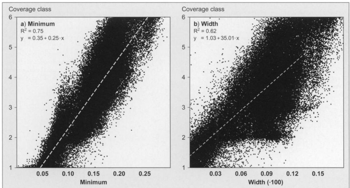
Fig. 6: Relationships between woody coverage and minimum (a) and width (b) of the parabolic curve fit Zusammenhang zwischen Gehölldichte und Parabelminimum (a) bzw. Parabelbreite (b)
