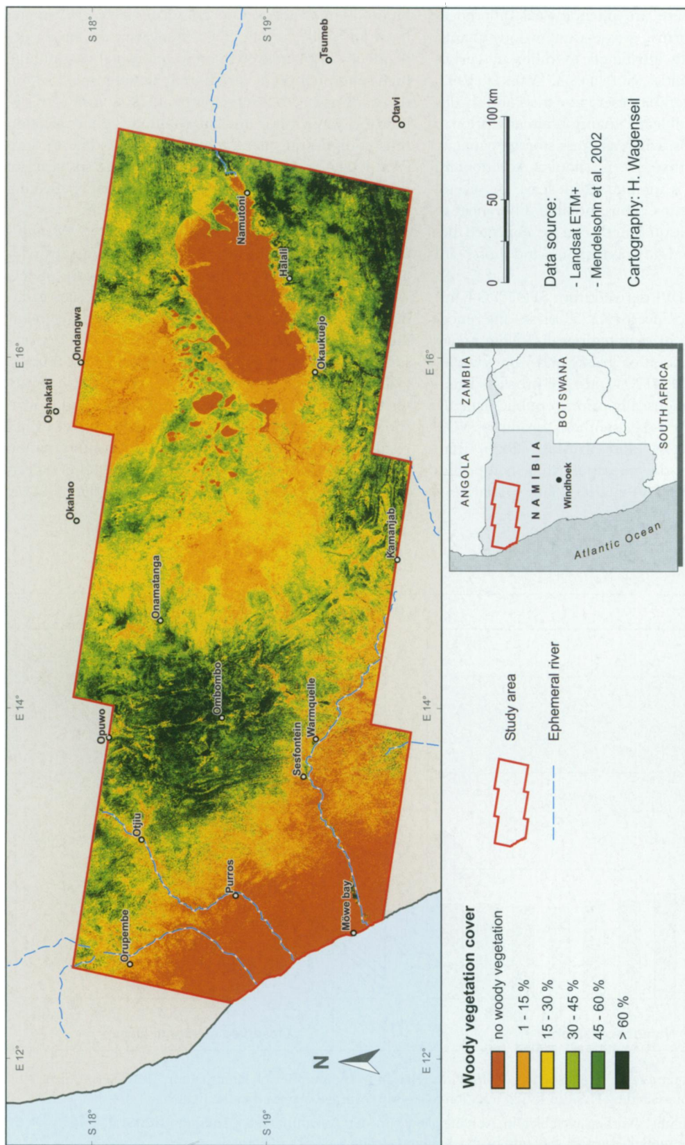
Fig. 3: Woody vegetation cover estimated from Landsat ETM+ Deckungsgrad der Gehölze, abgeleitet aus Landsat ETM+
