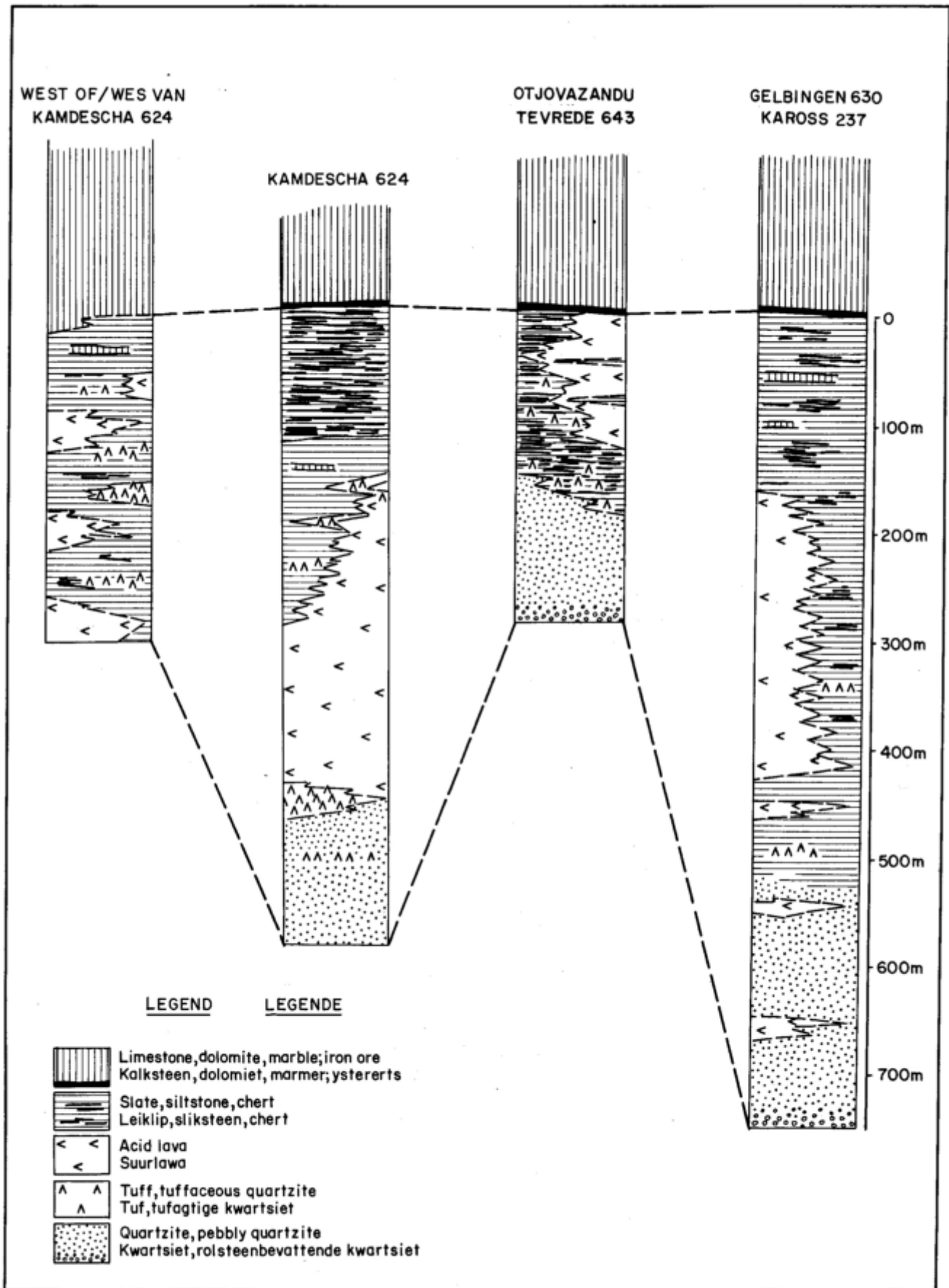
FIG. 1.— Section across the type area of the upper part of Otjovazandu Member of the Khoabendus Formation Snit oor die tipegebied van die boonste gedeelte van die Otjovazandudeel van die Formasie Khoabendus
