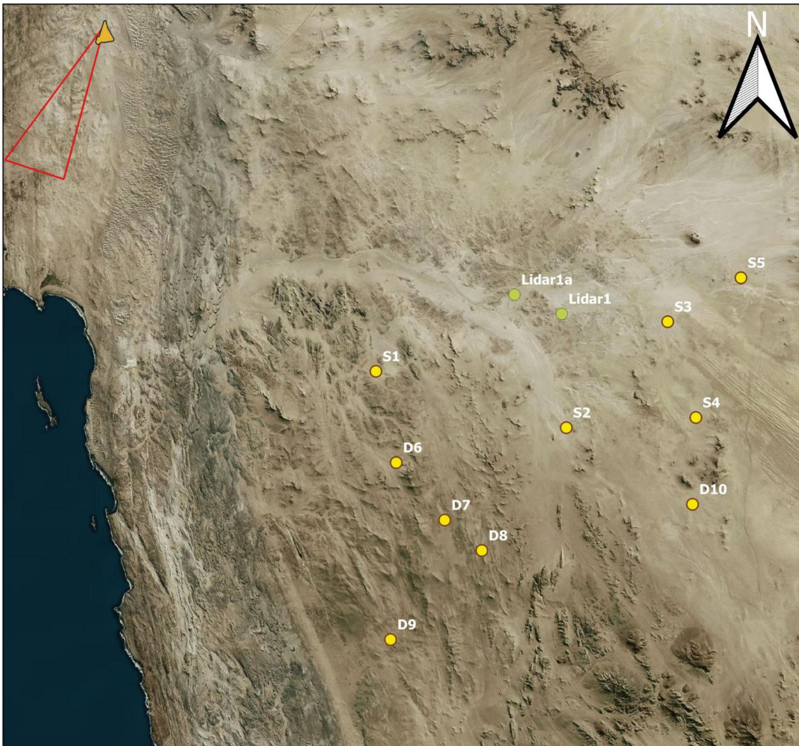
Lidar and Met Mast Locality Map
